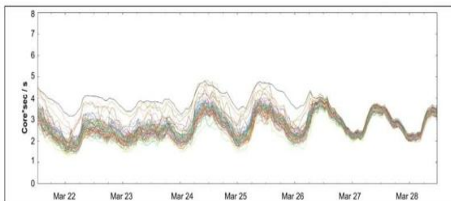
图20-6: 在启用加权轮询策略前后的CPU分布图
