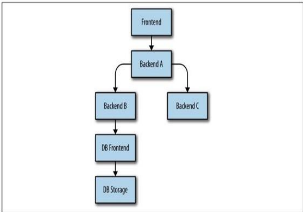
图21-2：某个依赖栈
