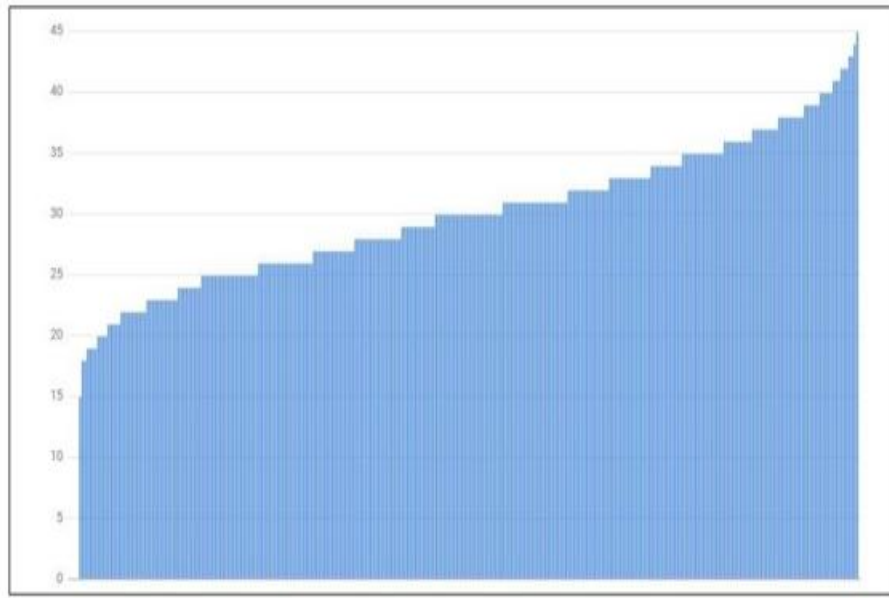
图20-4:300个客户端、300个服务器端和子集大小为10% 的连接分布图
