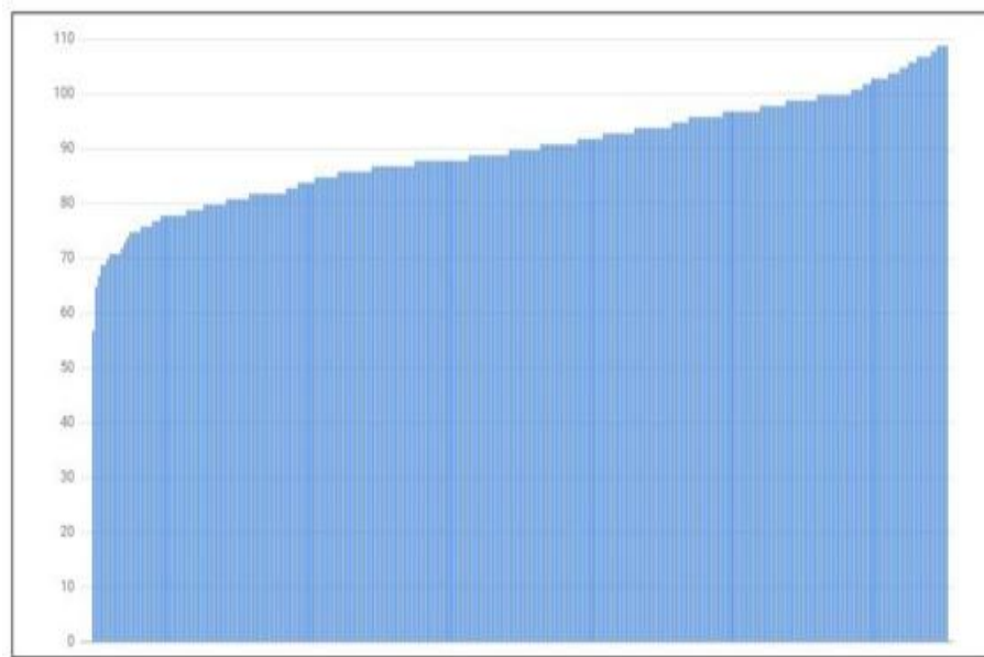
图20-3: 300个客户端、300个后端和子集大小为30%的连接分布图
