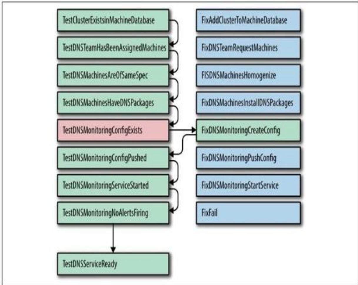
图7-2:DNS 服务的ProdTest，体现了一个失败测试的后果仅仅是多运行一个修复程序。左侧是测试，右侧是对应的修复程序。
