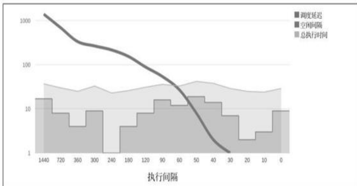
图25-1：周期性流水线执行间隔时间与等待时间（对数级Y轴）
