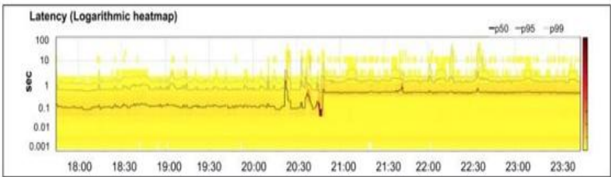
图12-4：应用程序延迟图，显示出50%、95%、99%请求的延迟（以线表示），同时用热力图显示了在指定时间内请求的分布情况。
