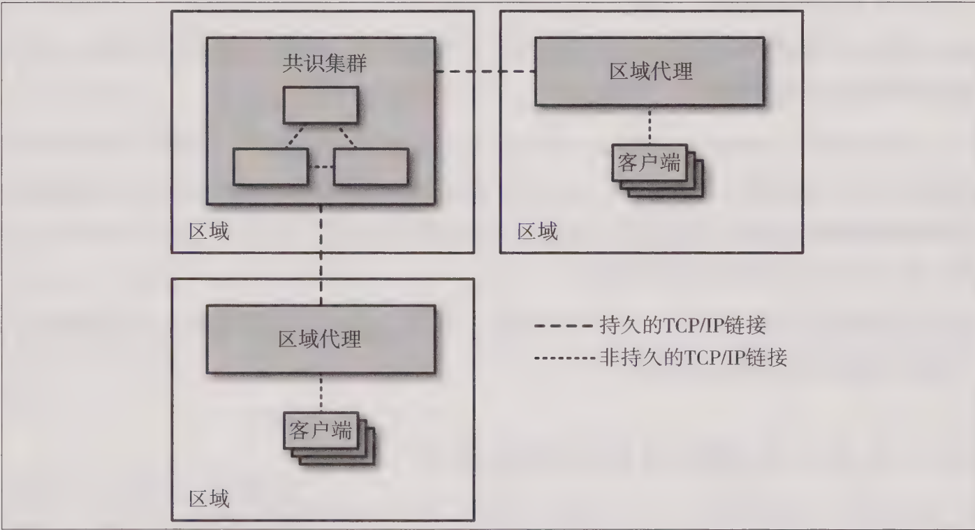
图23-9： 使用代理池来降低客户端跨地理区域打开TCP/IP连接的开销
