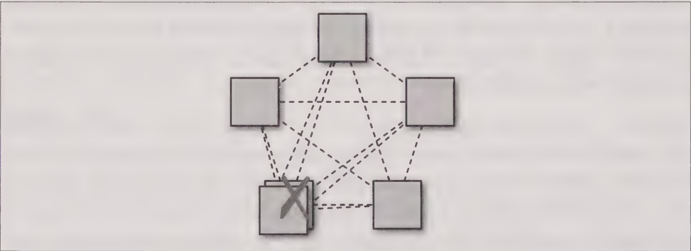
图23-10：向系统中一个区域增加一个额外的副本可能会影响系统可用性。 将多个副本放在同一个数据中心中可能会减少系统可用性：这里展示了当该数据中心出现故障时整个共识组没有任何备用副本可用。
