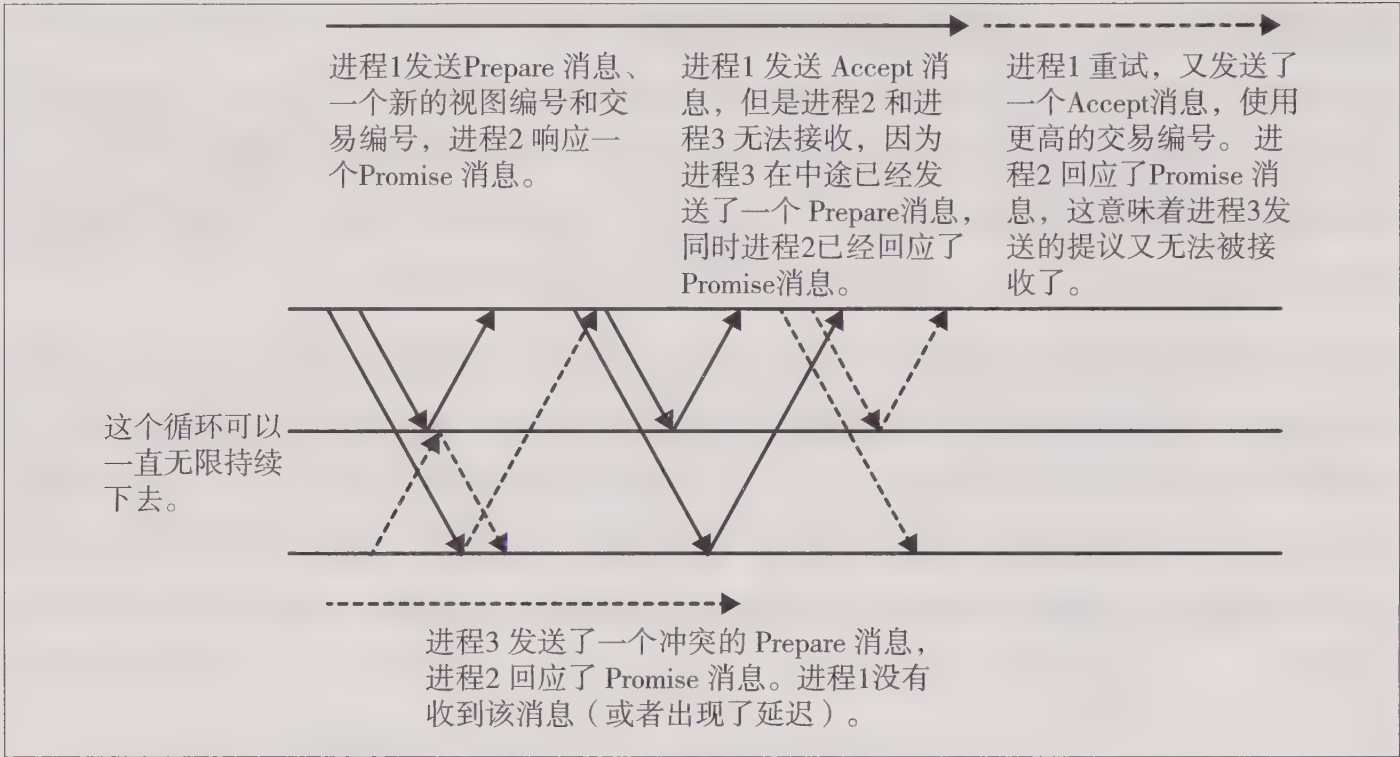
图23-8：复合Paxos协议中的“提议者决斗”场景
