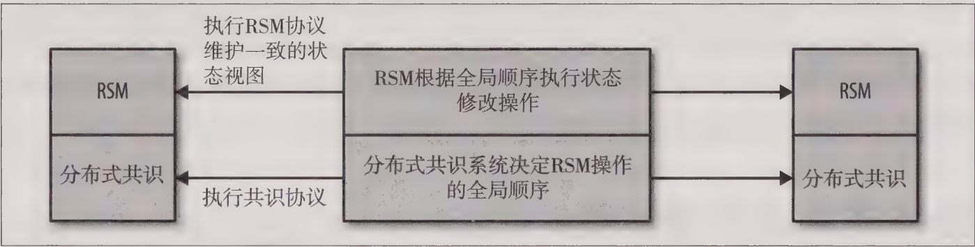
图23-2：共识算法和复制状态机的关系
