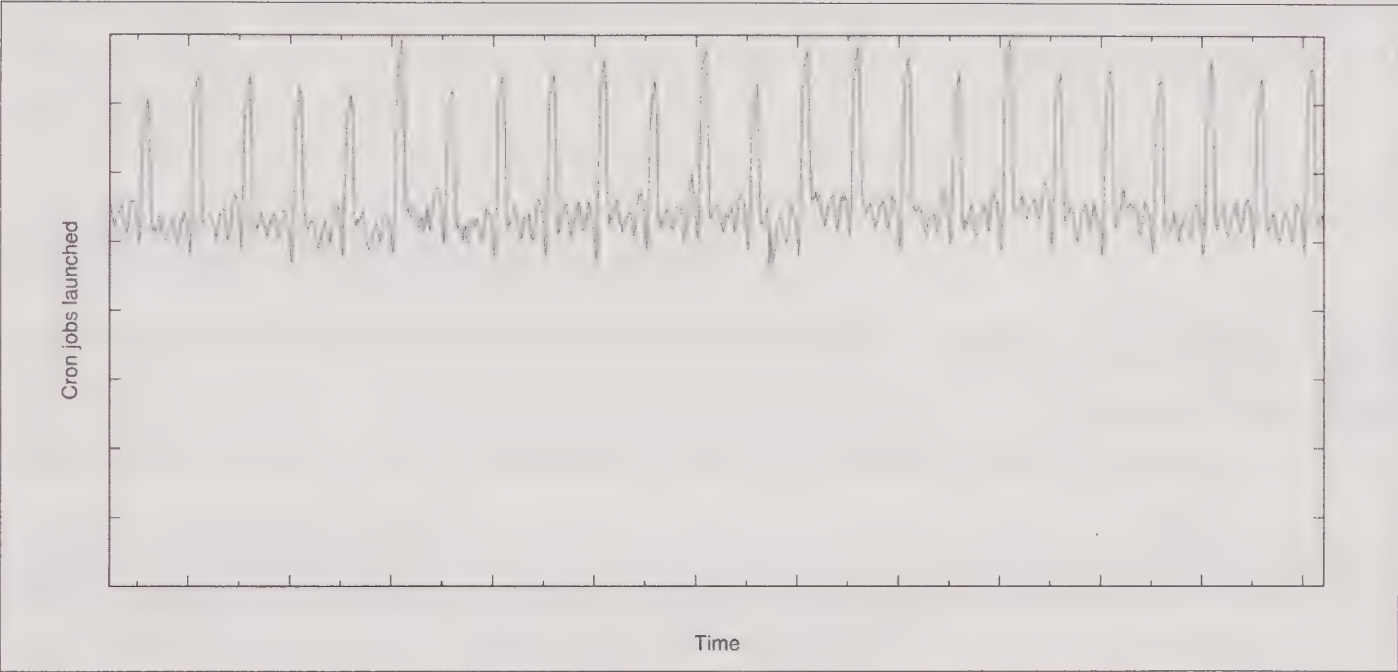
图24-3: 全球Cron任务的启动数量
