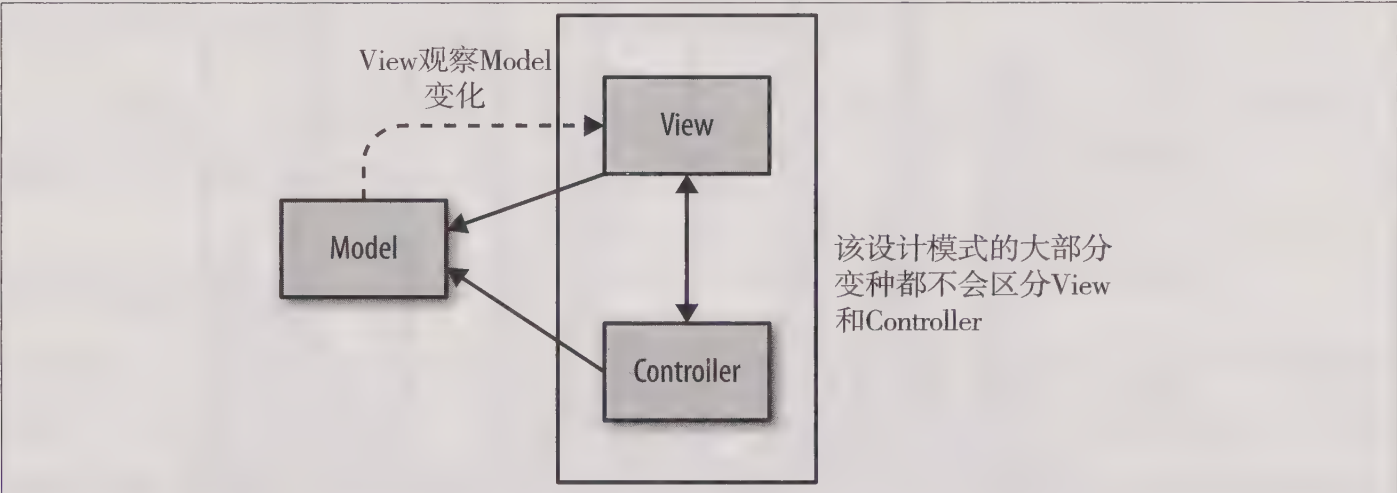
图25-4： 用户界面设计中常见的MVC模式
