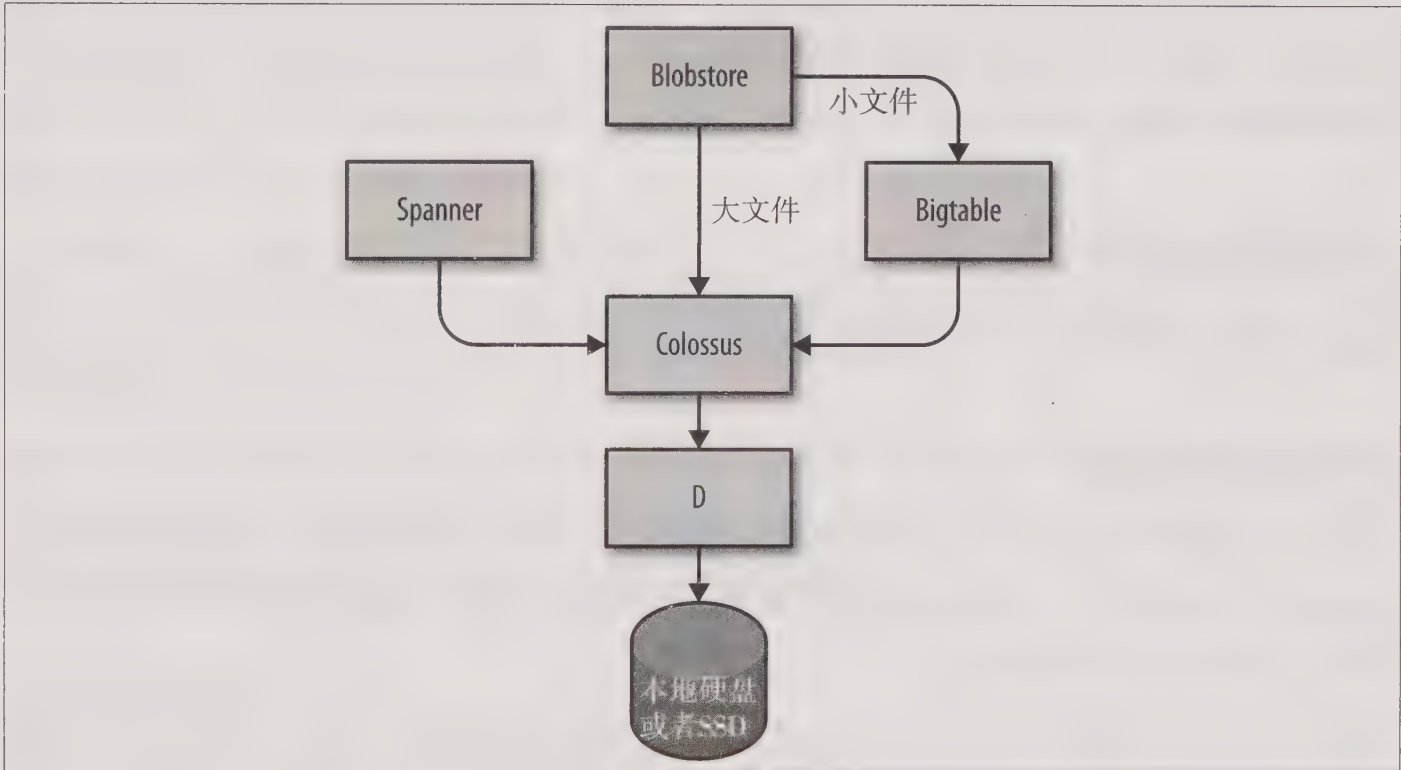
图2-3: Google 存储系统 (部分)
