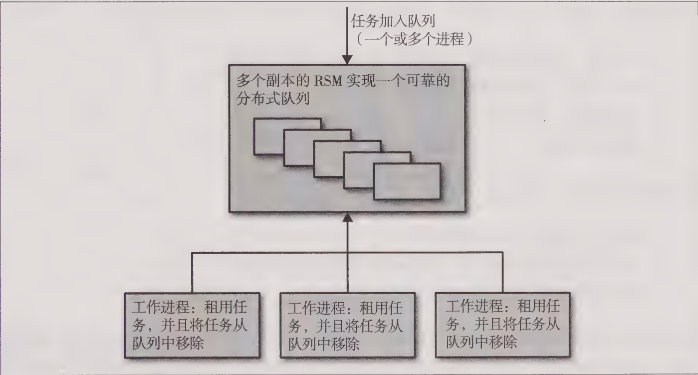
图23-5：一个基于队列的任务分发系统，利用分布式共识搭建的可靠队列。
