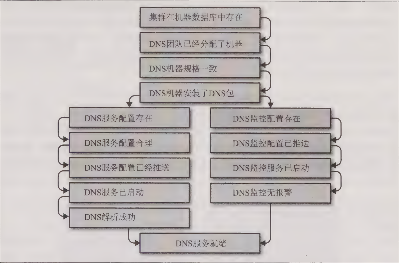
图7-1: DNS服务的 ProdTest，展示了一个测试出现问题后如何中止之后的一系列测试。
