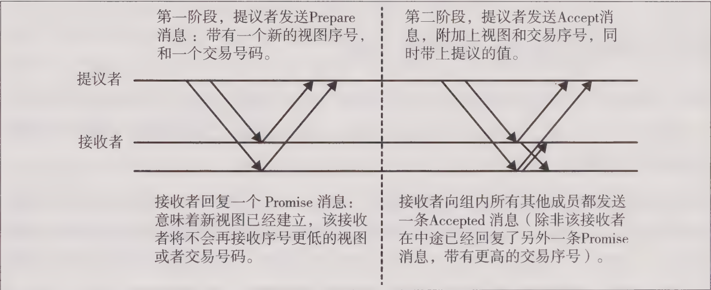
图23-7: 基本的复合式Paxos 消息流
