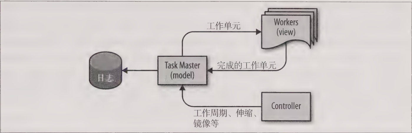
图25-5: Google Workflow系统采用的MVC模式
