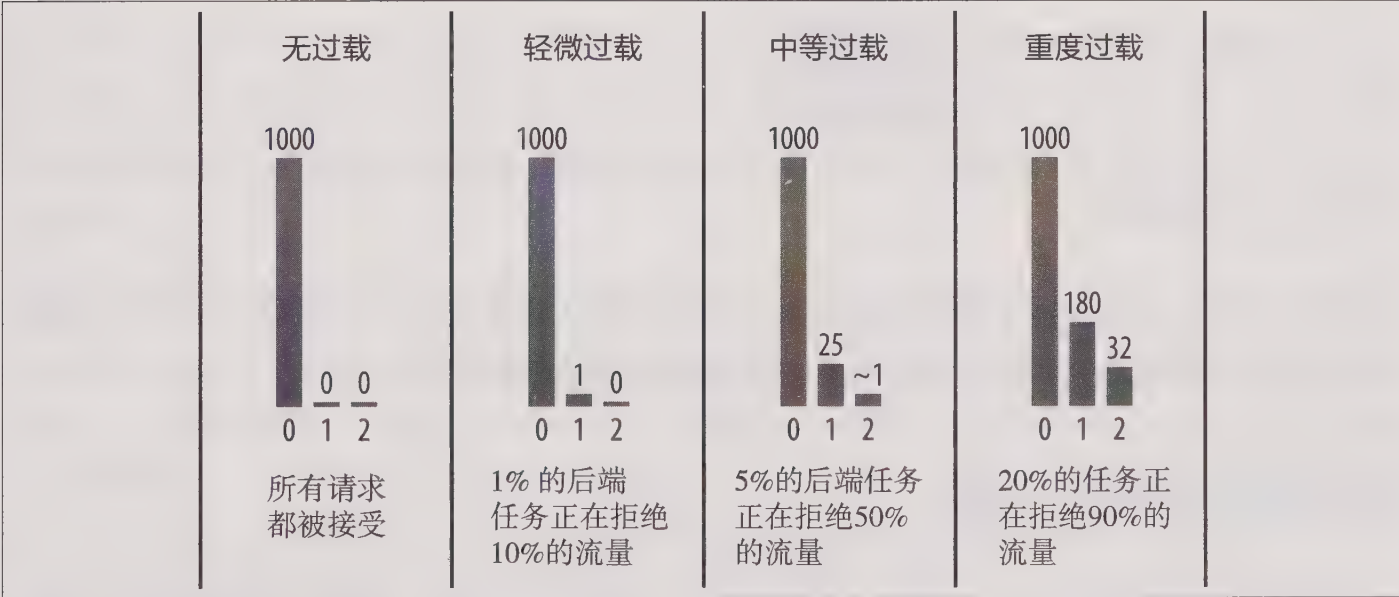
图21-1：不同情况下的请求直方图
