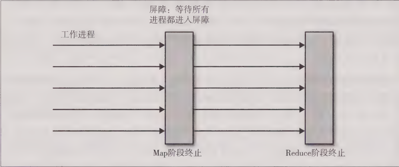
图23-4：在MapReduce计算中使用屏障协调进程
