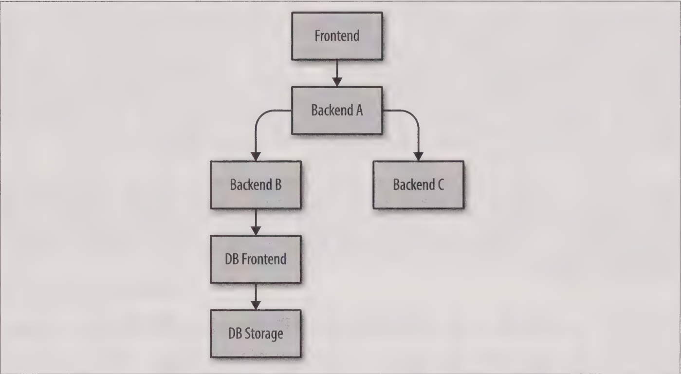
图21-2：某个依赖栈
