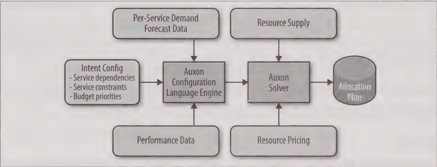
图18-1: Auxon的主要组件
