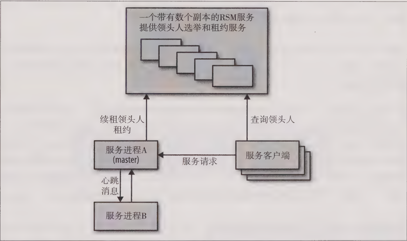
图23-3: 使用复制进程进行领头人选举构造的高可用系统
