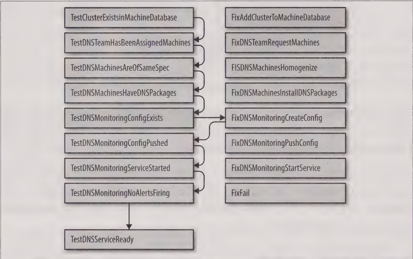
图7-2: DNS 服务的ProdTest，体现了一个失败测试的后果仅仅是多运行一个修复程序。左侧是测试，右侧是对应的修复程序。
