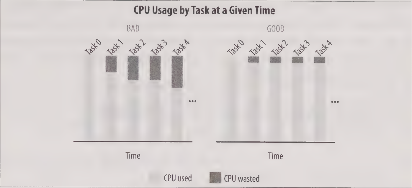
图20-2: CPU的使用和浪费的直方图
