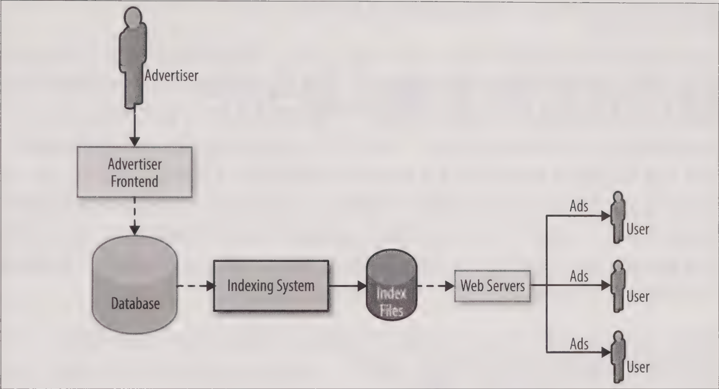
图31-1：一种通用的广告服务系统
