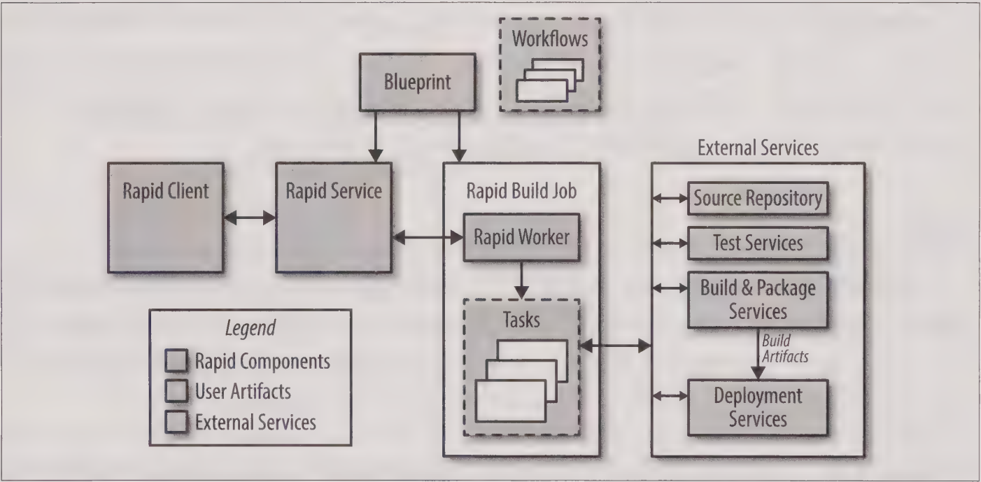
图8-1：简化版Rapid架构，展示了系统的主要组件。
