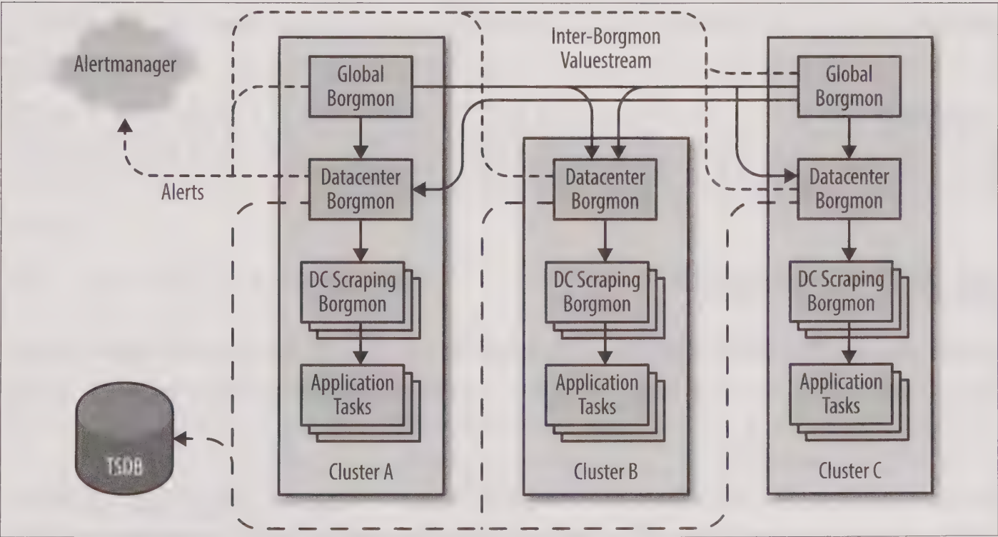
图10-3: 一个在三个集群中层级部署的Borgmon 数据流向图
